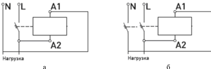
Рис. 2 – Схемы включения расцепителей минимального напряжения, максимального напряжения, минимального и максимального напряжения, выполненного в общем корпусе: а – с однополюсным автоматическим выключателем, б – с двухполюсным автоматическим выключателем.
