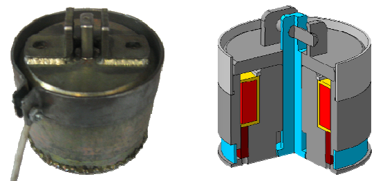
Рис. 5 Поляризований моностабільний електромагніт
