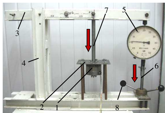
Рис. 6 Стенд для визначення сили притискання яркіря до нерухомої частини магнітопроводу
