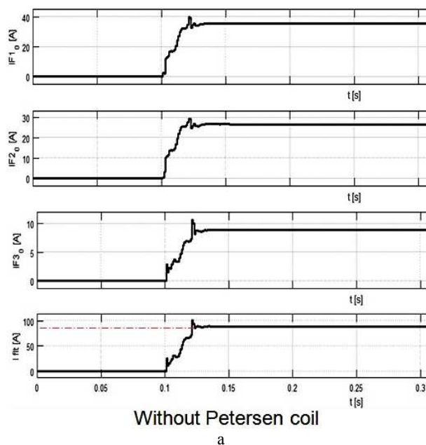
Рис. 14. Режим ОЗЗ. Сравнение осциллограмм аварийных токов и токов нулевой последовательности фидеров в сетях: а – с изолированной нейтралью; б – компенсированной катушкой Петерсена нейтралью
