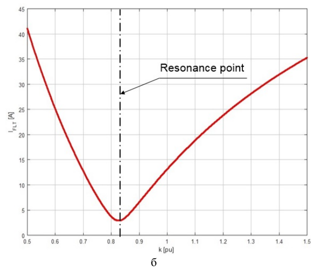
Рис. 15. Графики зависимостей аварийного тока от различных уровней компенсации катушки Петерсена: а – без учета влияния индуктивности рассеяния вспомогательного трансформатора; б – с учетом влияния индуктивности рассеяния вспомогательного трансформатора
