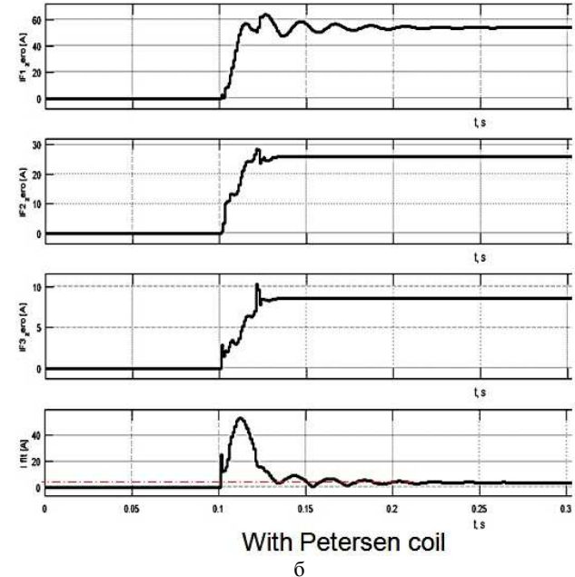
Рис. 14. Режим ОЗЗ. Сравнение осциллограмм аварийных токов и токов нулевой последовательности фидеров в сетях: а – с изолированной нейтралью; б – компенсированной катушкой Петерсена нейтралью
