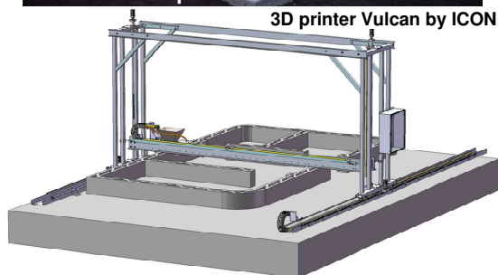
Рис. 14. Прототип 3D-друкованого будинку (зверху) та зовнішній вигляд 3D-принтеру Vulcan (знизу)
