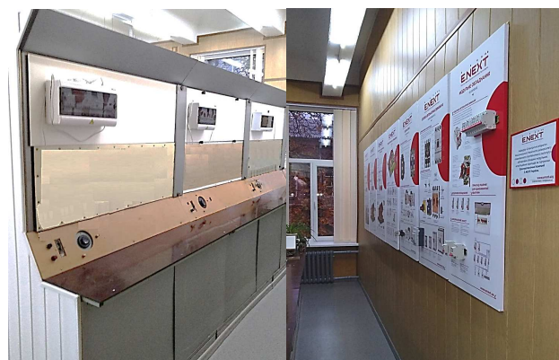
Рис. 13. Ряд лабораторних столів, обладнаних модульною комутаційною апаратурою компанії E.NEXT (ліворуч) та демонстраційні стенди цієї компанії (праворуч)
