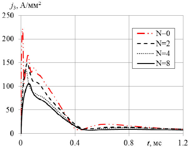
Рис. 4 – Усредненные плотности токов в ФЭ, выполненном с N радиальными разрезами
