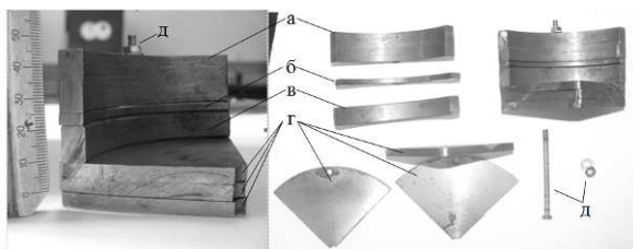
Рис. 11 – Элементы четверти составного ФЭ
