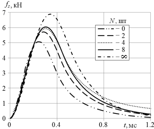
Рис. 6 – Электродинамические усилия, действующие на якорь ЛИДП в зависимости от количества N радиальных разрезов ФЭ
