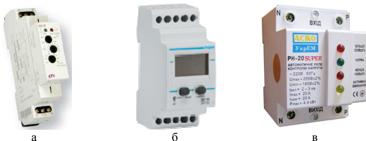
Рис. 1 – Примеры реле напряжения модульного исполнения: а – реле HRN-33 (-35) [1] (ETI, Словения), б – реле EU-102 [2] (Hager, Германия), в – реле серии PH-S [3] (AcKo-УКРЕМ, Украина).
