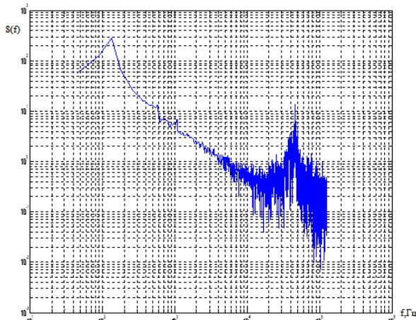
Рис. 2 – Спектр сигнала измерительной обмотки
