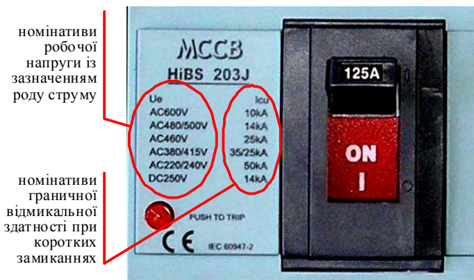
Рис. 4 – Лицьова панель апарата захисту від коротких замикань, на якій виробник розмістив номінативи граничної відмикальної здатності цього апарата при коротких замиканнях ( I_{cu} ) залежно від роду струму (AC / DC) та номінативу робочої напруги ( U_e )
